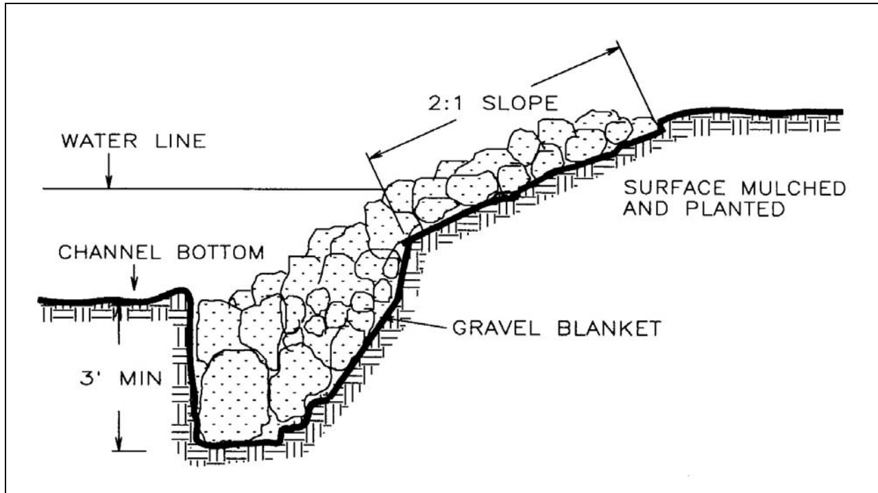
Figure VII-48. Riprap.
